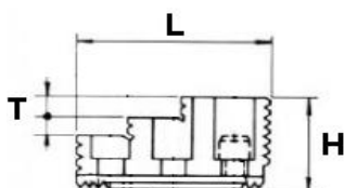
Gehärtete umkehrbare Stufenbacken / Hard top reversible jaws step type
